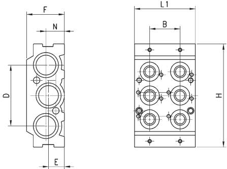
CNVL-3I2用於3系列G1/8電磁閥 CNVL-4I2用於3系列G1/4電磁閥
