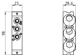
可安裝1個3系列G1/8電磁閥
