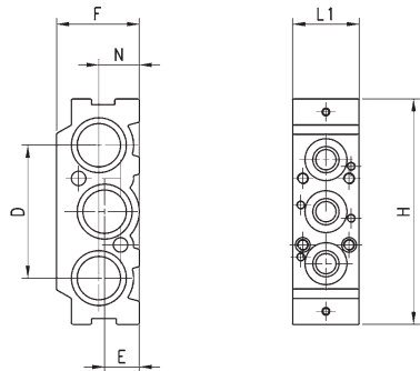
CNVL-3I1用於3系列G1/8電磁閥 CNVL-4I1用於3系列G1/4電磁閥
