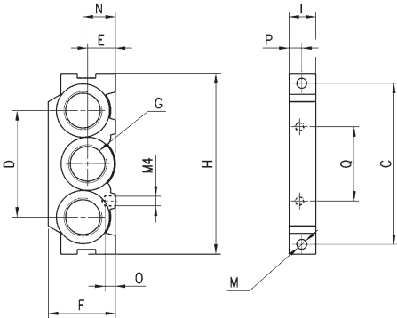
CNVL-3H用於3系列G1/8電磁閥 CNVL-4H用於3系列G1/4電磁閥
