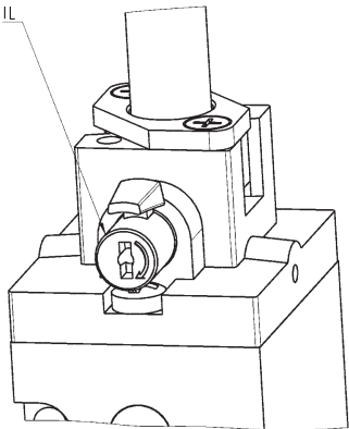
IL：槓桿式手控裝置，雙穩式
