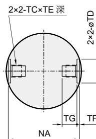
A-A 剖面
